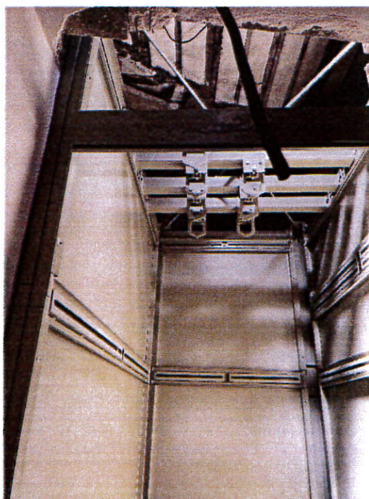
Colocación de estructura portante:
